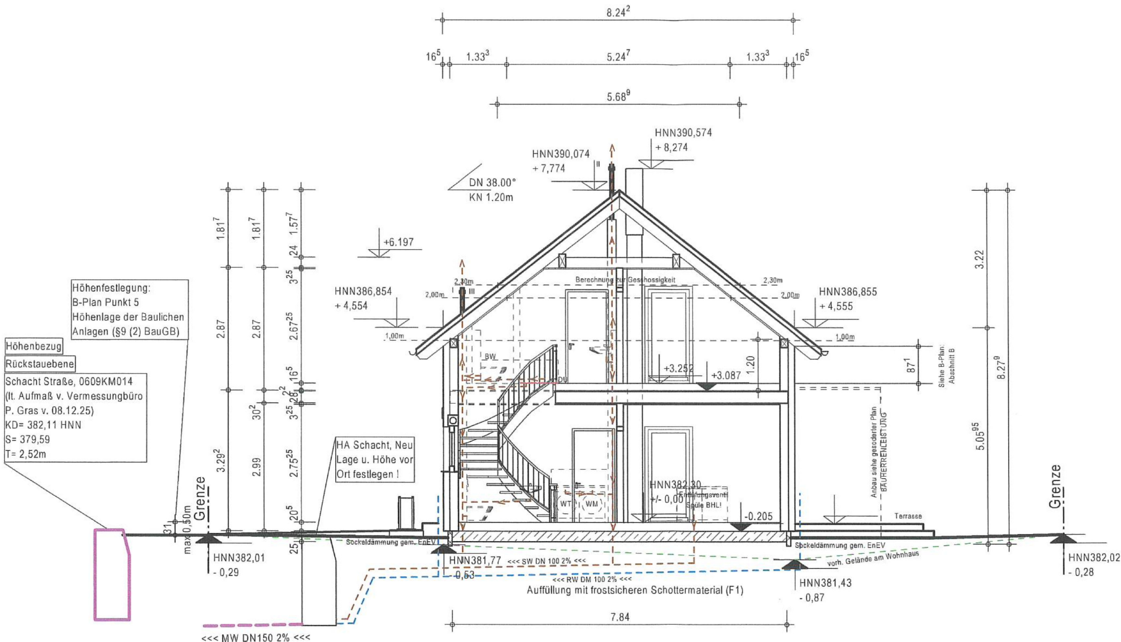
Querschnitt M 1:100
