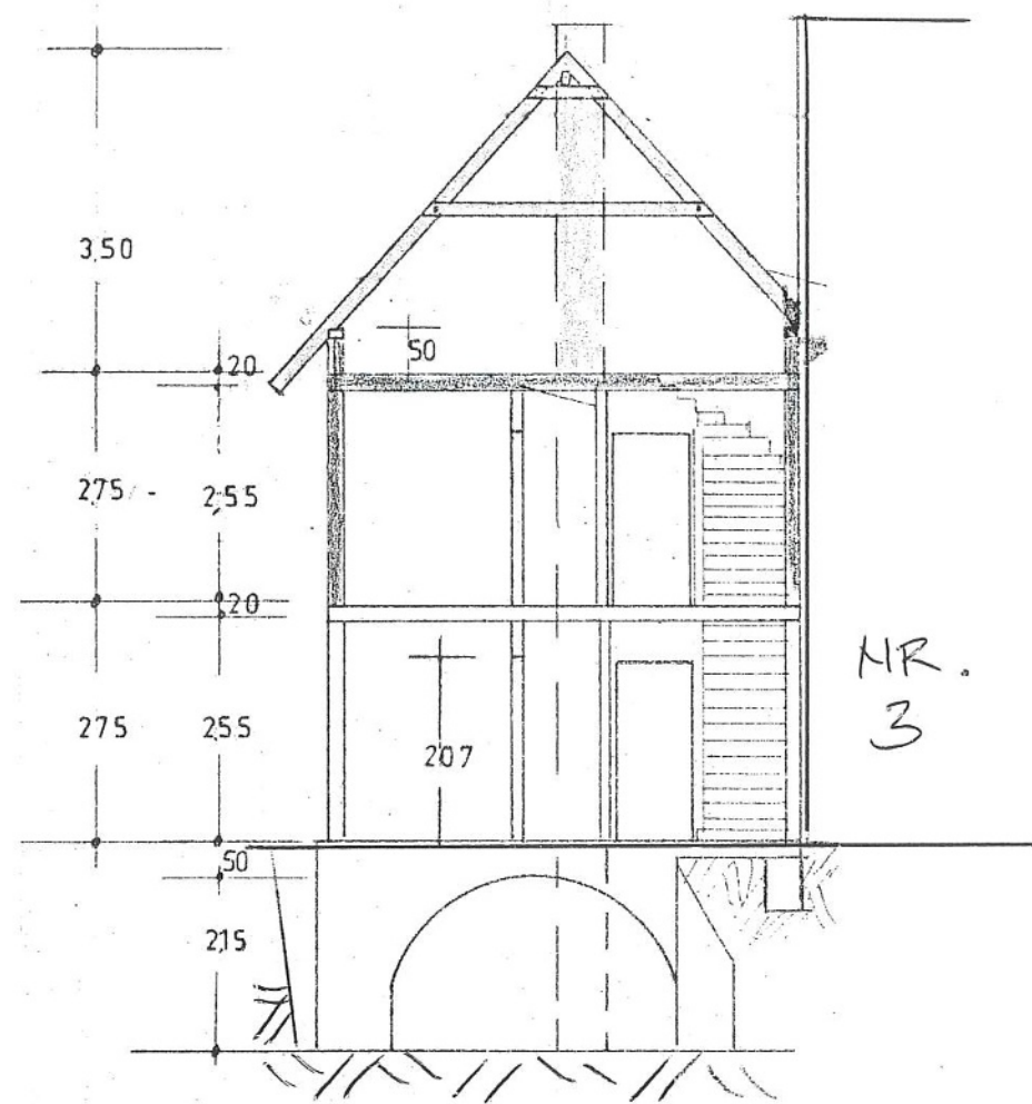
SCHNITT A-B UNVERÄNDERT
