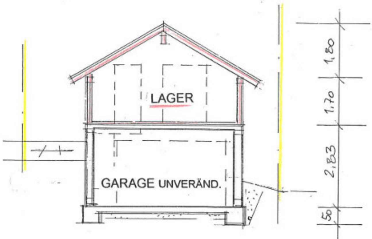
SCHNITT A-A
