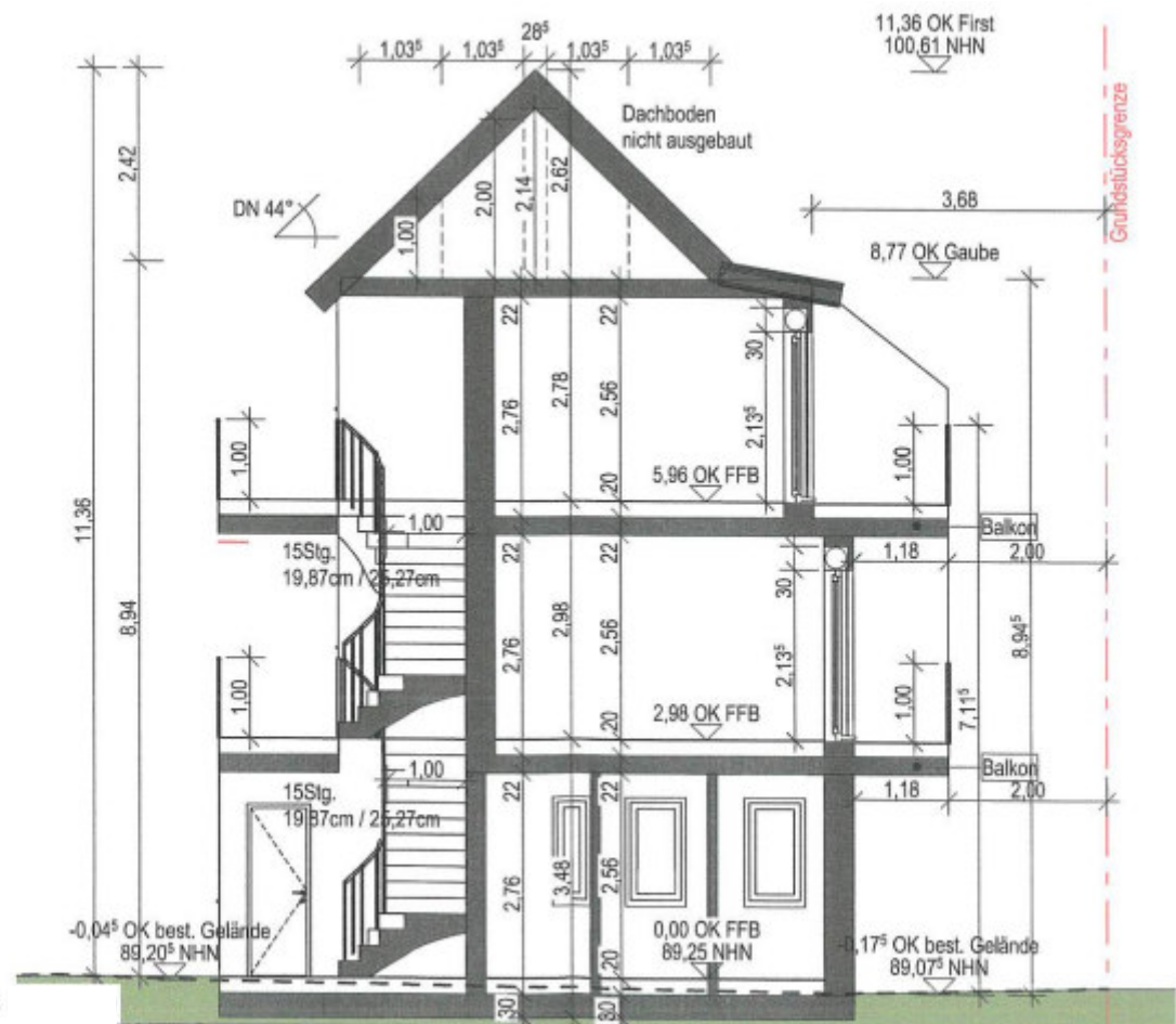
Schnitt B-B
