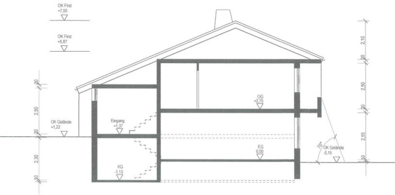
Schnitt B_B
