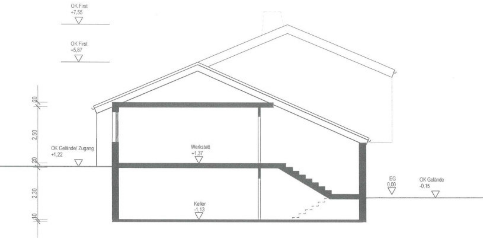
Schnitt A_A
