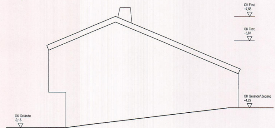
Ansicht Ost
