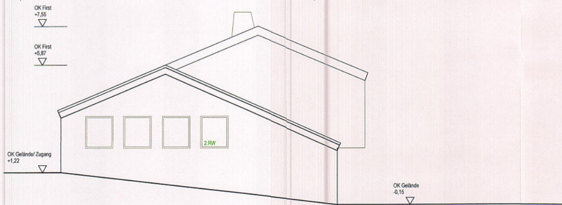
Ansicht West
